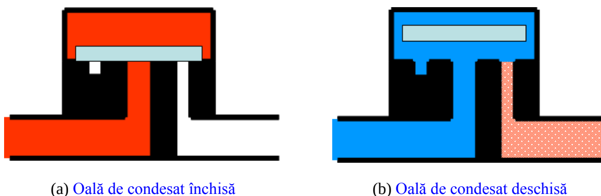
Figura 27: Funcționarea tipului termodinamic de separare a condensatului (Sursa: US DOE Steam BestPractices End User Training)
