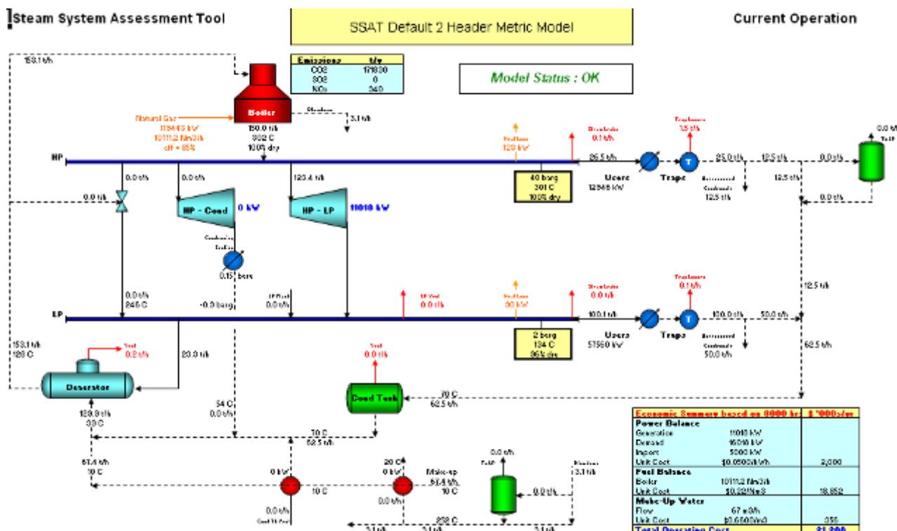
Figura 43: Exemplu –Modelul Sistemului de Abur
