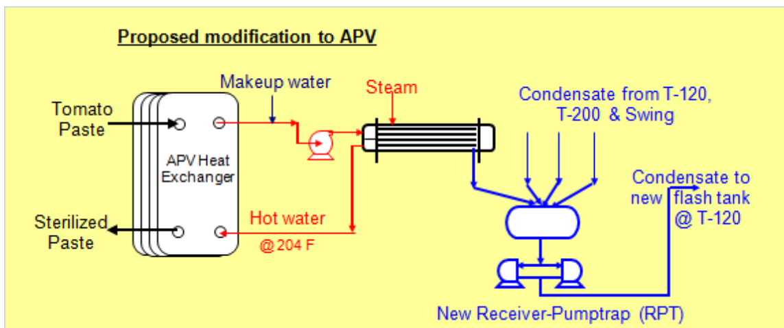
Figura 47: Procesul schematic de curgere a îmbunătății sistemului de vaporizatoare “Paste Sterilizer”
