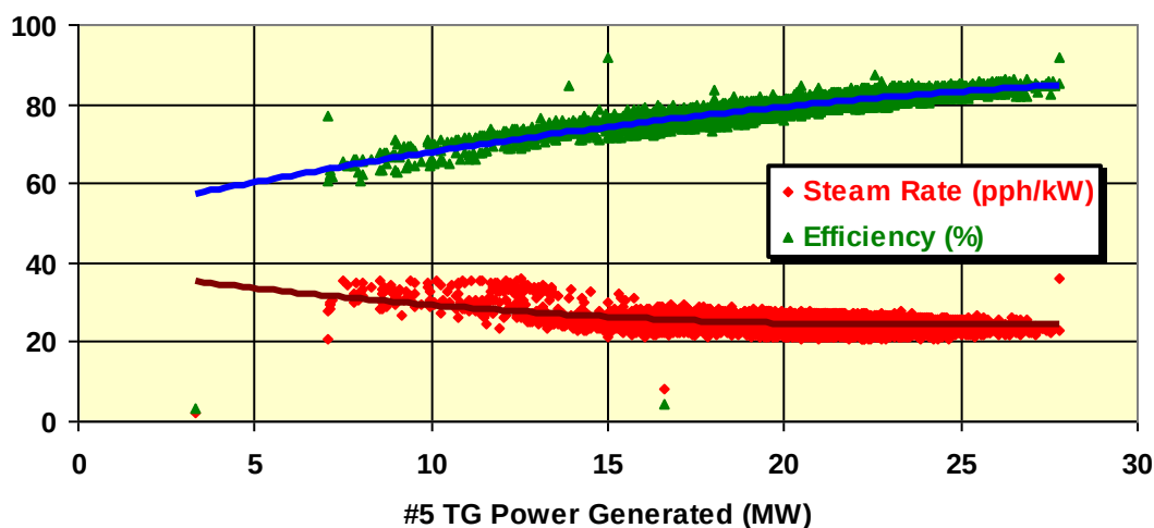
Figura 42: Exemplu – Curba de eficiență a operării turbinei cu abur
