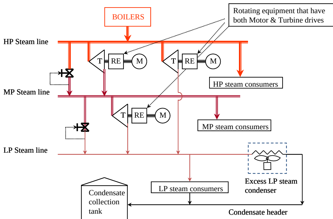
Figura 48: Diagrama Bilanțului Sistemului de Abur la o Rafinărie
