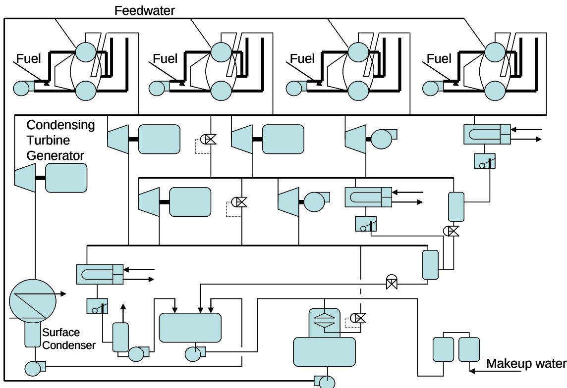
Figura 2d: A 3- Diagrama sistemului de abur cu turbină de condensat la presiune înaltă (Sursa: US DOE Steam BestPractices End User Training Program)
