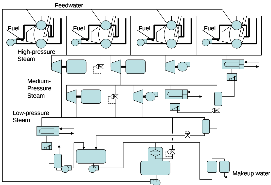
Figura 2c: A 3- Diagrama sistemului de abur la presiune înaltă (Sursa: US DOE Steam BestPractices End User Training Program)
