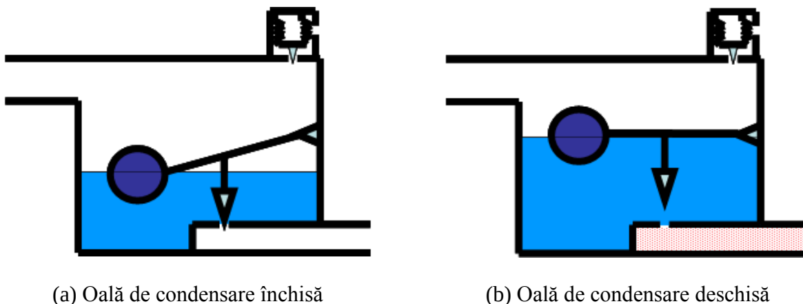
Figura 25: Func ionarea mecanic  a separatorului de condensat din abur (Sursa: US DOE Steam BestPractices End User Training)
